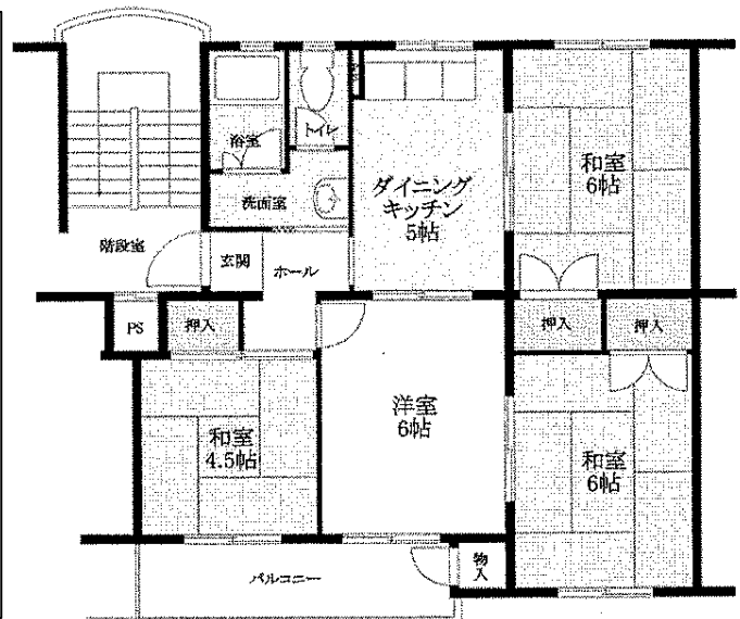
間取図
